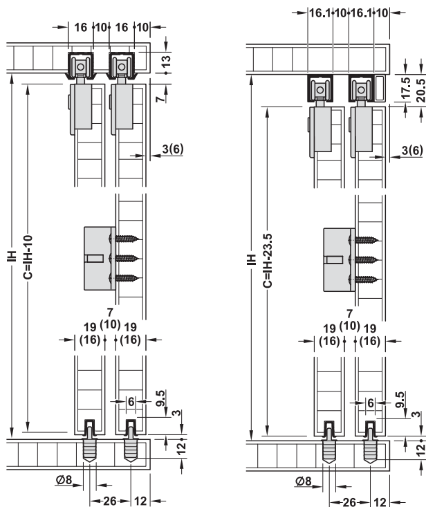
szyna górna wpuszczana
