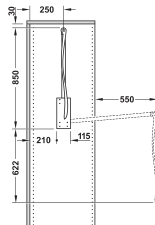
montaż na środku ściany bocznej korpusu
