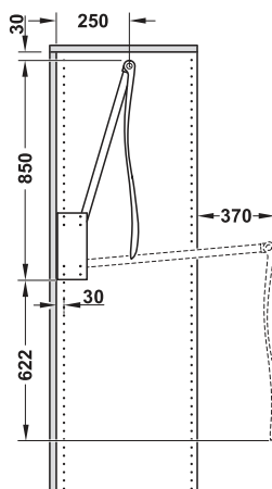
montaż w tylnym rzędzie otworów
