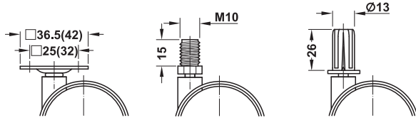
Anschraubplatte
