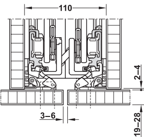
Parktasche für 2 Türflügel, Breite 110 mm
