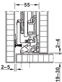
Parktasche für 1 Türflügel, Breite 55 mm
