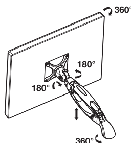
Schwenkarm mit mittlerem Arm
