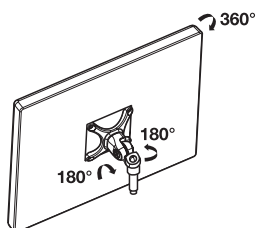
Schwenkarm mit kurzem Arm
