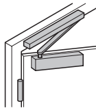
Normalmontage Bandseite
