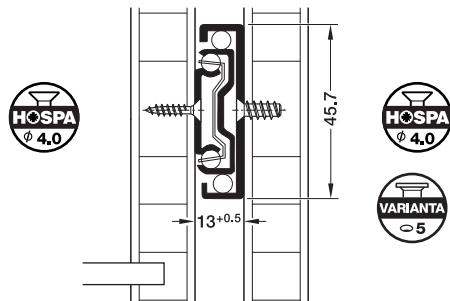
seitliche Montage
