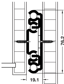
Accuride 9301 und 9308 seitliche Montage
