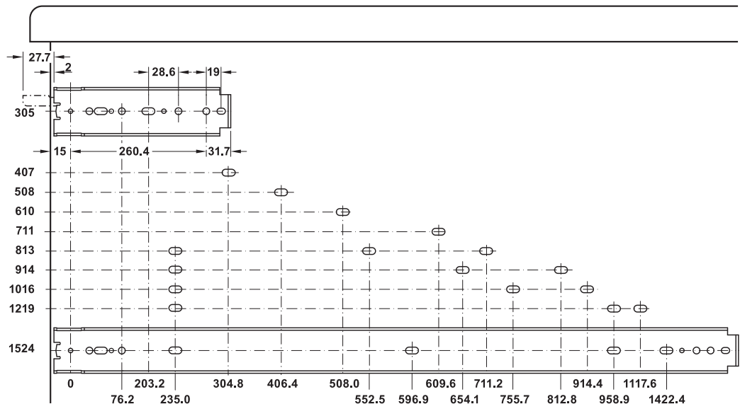
Accuride 9301 aufliegende Montage
