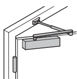
Normalmontage auf der Bandseite
