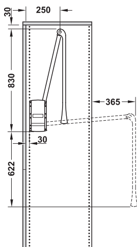
Einbau hintere Lochreihe
