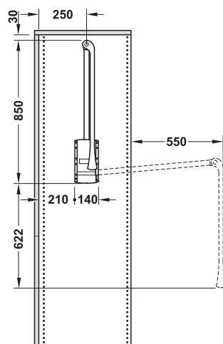
Einbau Mitte Schrankseitenwand
