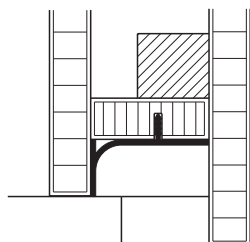
przykład montażu
