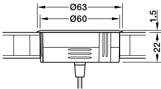
Montaż nawierzchniowy
