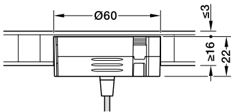
Montaż ukryty
