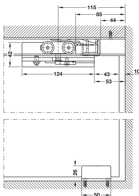
Schnitt Rollenwagen und Bodenführung
