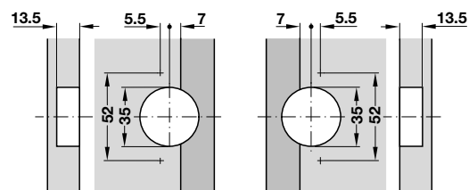
Schemat wierceń, kąt uciosu 45°
