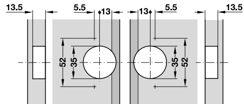
Schemat wierceń, kąt uciosu 22,5°
