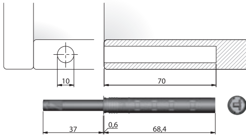
Schemat wierceń dla wersji wpuszczanej
