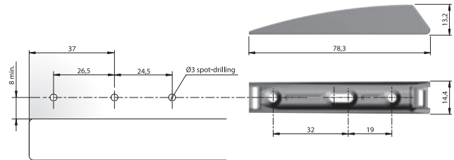
Schemat wierceń i wymiary adaptera dla wersji 37 mm
